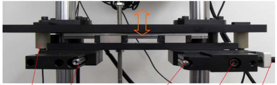
스토퍼 직경측정Tip 기준핀 가이드고정나사 직경조정나사
